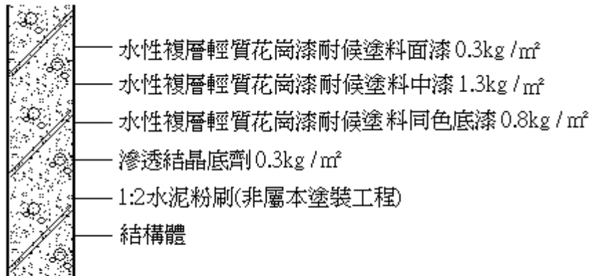
外牆水性複層輕質花崗漆耐候塗料塗裝工程施工圖
